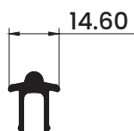
U-Guiderail
