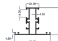
T-Mullion
