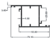
Inward Shutter (Big)
