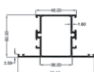
Big T-Mullion
